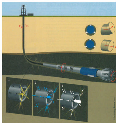
Grafik 1: Horizontale Bohrung (Quelle: Technology Review 10/2010)
